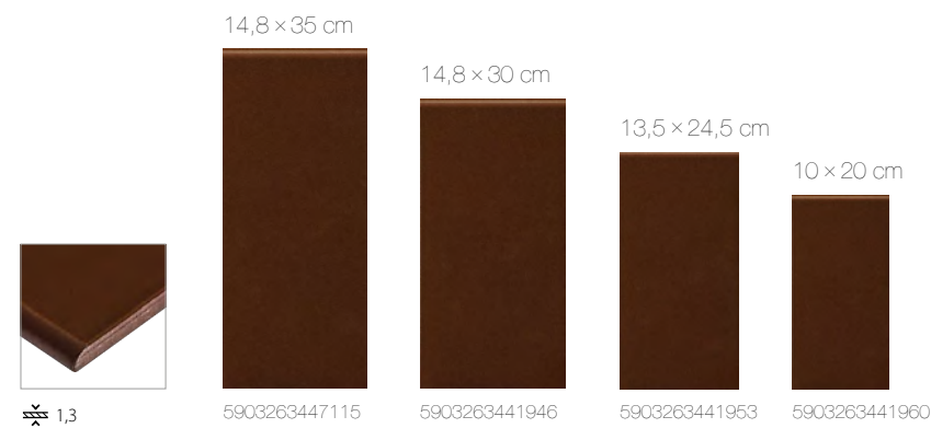
Brazowa płytka parapetowa szklwiona / подоконник глазурованный / глазурована плитка для підоконня
